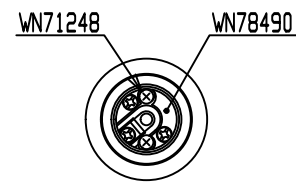
D(1:3) ソケット取付け
