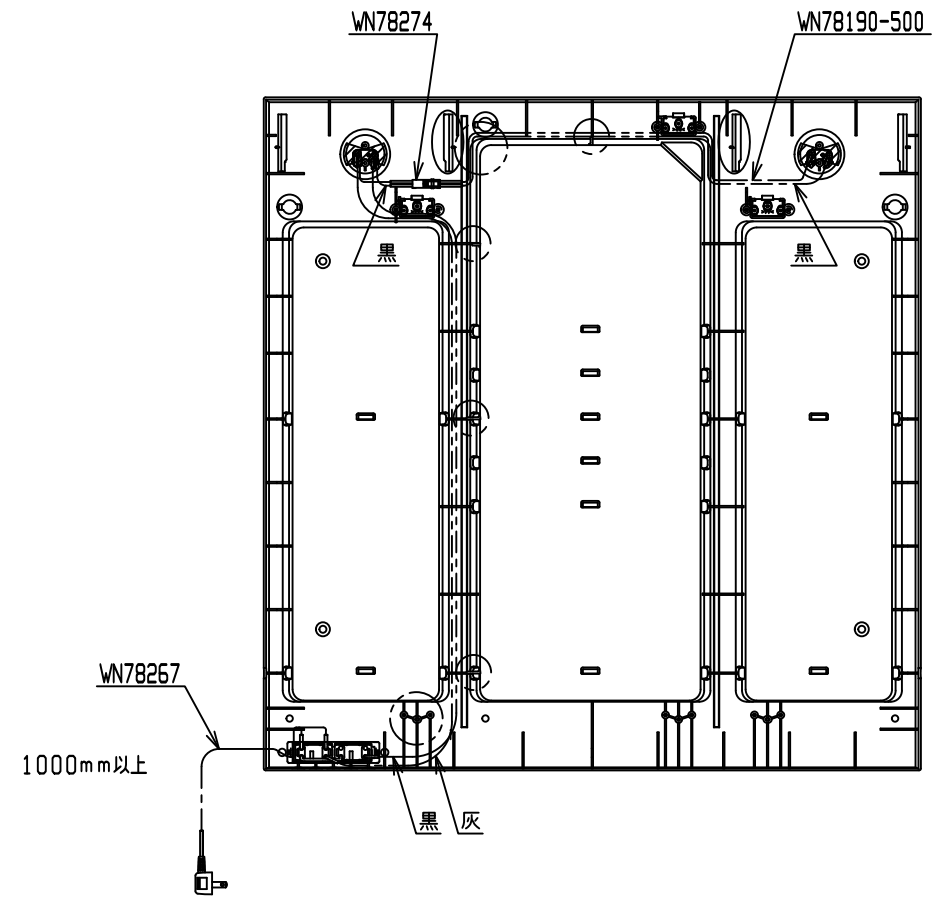
裏面図
