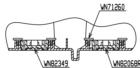
B-B(1:3)
